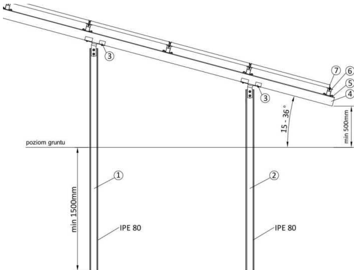
Rysunek. Szczegół konstrukcji dwupodporowej.
