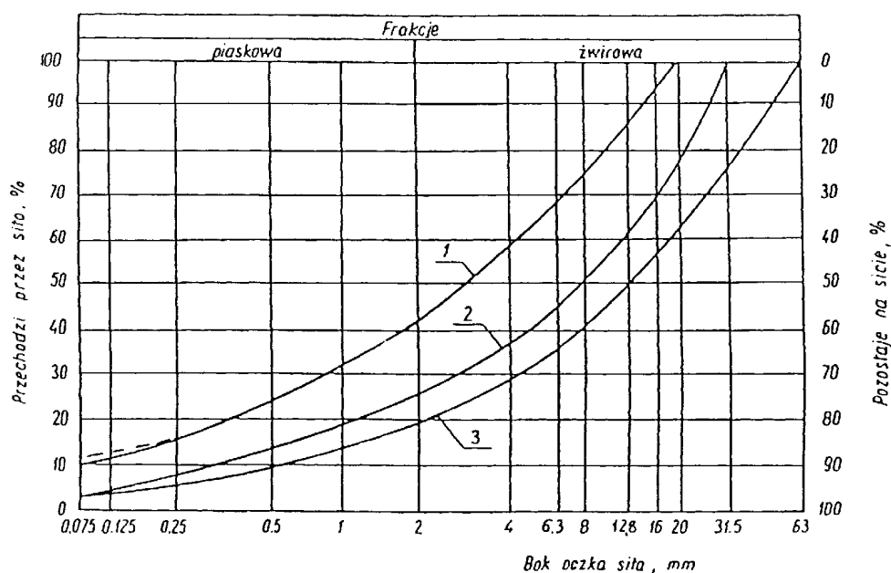
Rysunek 1. Pole dobrego uziarnienia kruszyw przeznaczonych na podbudowy wykonywane metoda stabilizacji mechanicznej 1-2 kruszywo na podbudowie zasadnicza (górną warstwą) lub podbudowę jednowarstwową 1-3 kruszywo na podbudowie pomocnicza (dolną warstwą)
